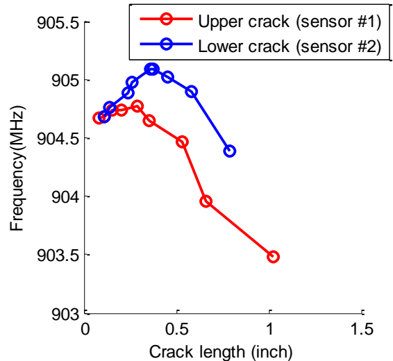
(d) Resonance frequency versus crack length
