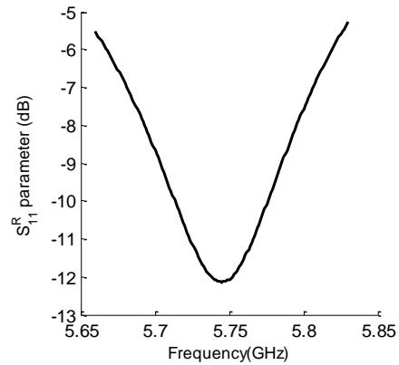
(b) Simulated S_{11}^R parameter
